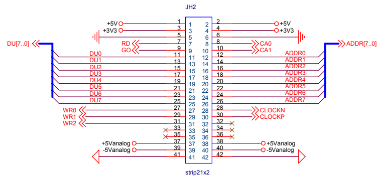
Connettore MB/moduli
